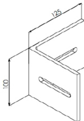
ANC 967 ANCORAGEM DA COLUNA A 90°
