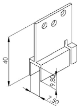
BX 003 GUIA DO BOX SISTEMA BX
