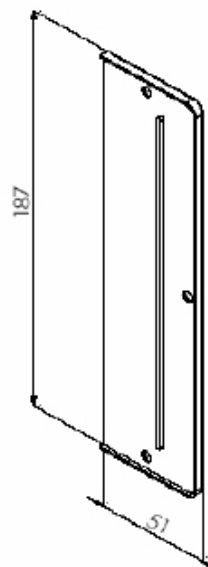
NYL 383 TAMPA DA INTEGRADA
