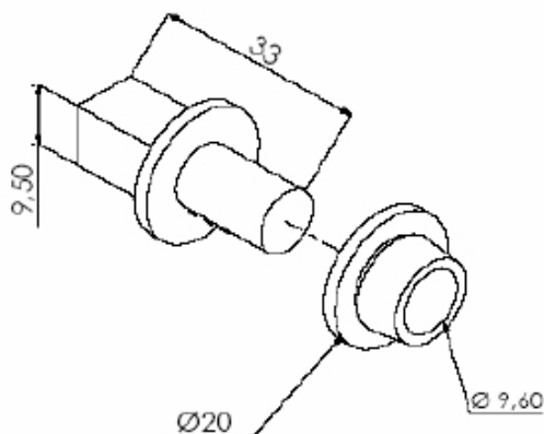
NYL 231 CONJUNTO PINO/BUCHA PARA BRISE
