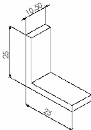
NYL 219 CANTONEIRA DE FECHAMENTO BOX ALUMÍNIO
