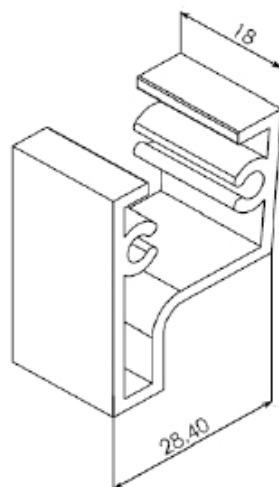
PRE 208 FIXADOR DA TRAVESSA LINHA FACHADA ATLANTA
