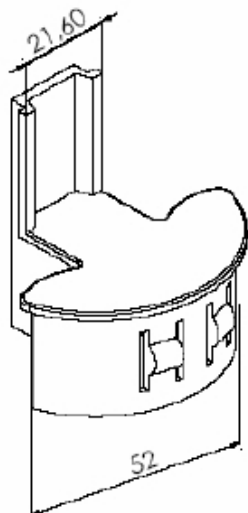
NYL 400A TAMPA DO MONTANTE LINHA D'ORO (ALUMIGON)
