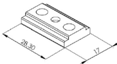
BX 004 CALÇO P/ BOX SISTEMA BX
