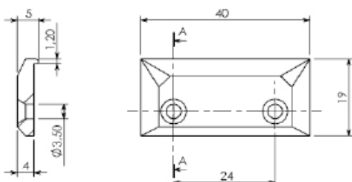
CON 063 CONEXÃO P/ CONTRA MARCO CN 063 E CN 200 C PARAFUSOS
