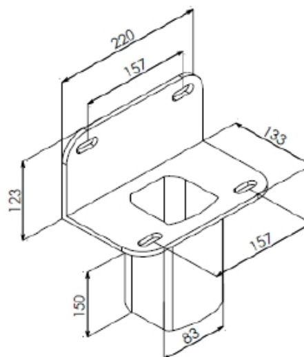
ANC 977 ANCORAGEM DE ALUMÍNIO
