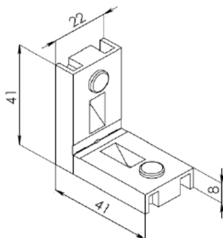
CON 377 MACHO DE CONEXÃO
