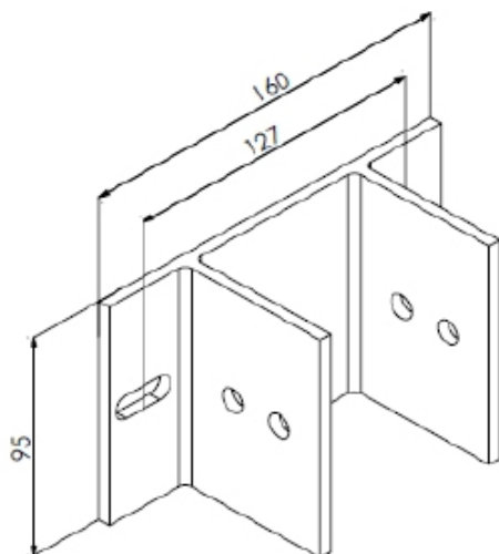
ANC 951 ANCORAGEM PARA COLUNA LINHA PV II E III
