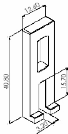
NYL 006 GUIA DESLIZANTE TRAVA FOLHA NYLON
