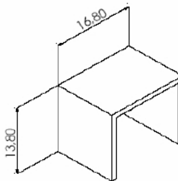
NYL 220 GUIA BRANCO DESLIZANTE INFERIOR BOX
