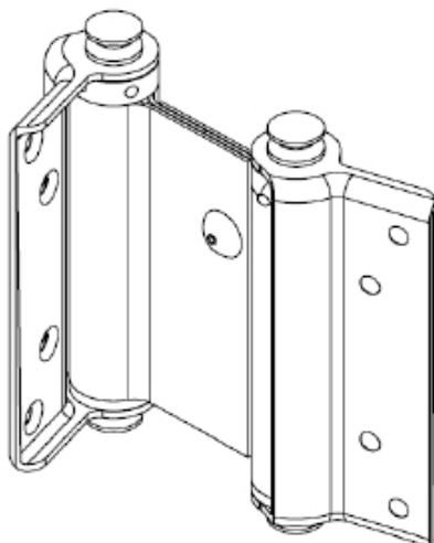
DOB 567 DOBRADIÇA VAI-VEM 4"
