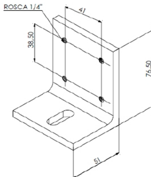
ANC 966 ANCORAGEM P/ COLUNA DE CANTO LINHA PV II E III
