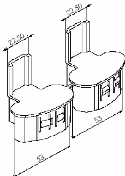
NYL 400 TAMPA P/ LG 021 DIREITO/ESQUERDO
