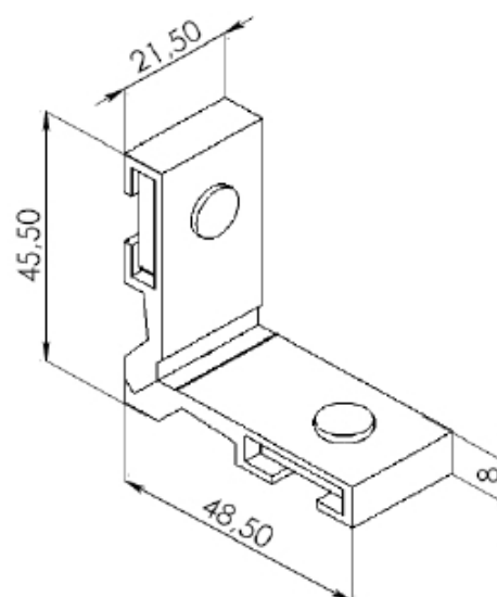
CON 377A MACHO DE CONEXÃO
