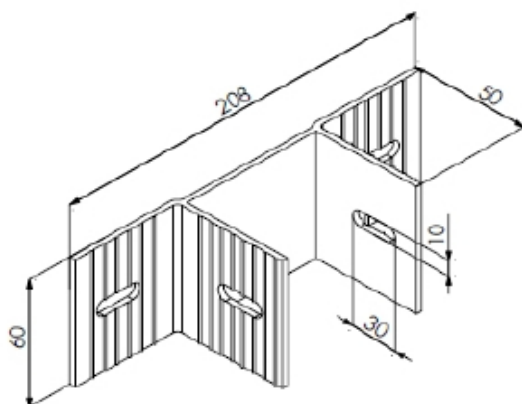
ANC 805 ANCORAGEM CENTRAL LINHA CITTÁ DUE
