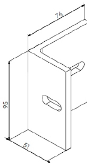
ANC 966 ANCORAGEM P/ COLUNA DE CANTO LINHA PV II E III
