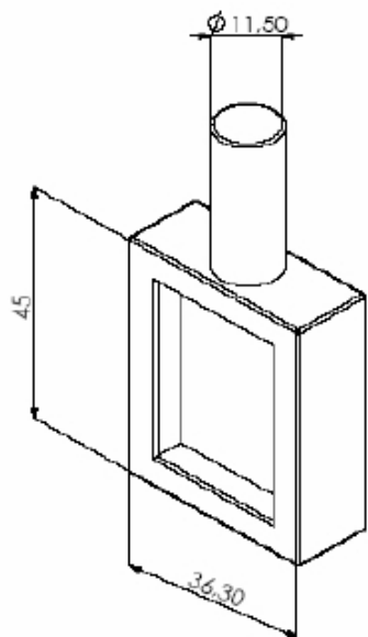
NYL 201 GUIA DESLIZANTE SUPERIOR
