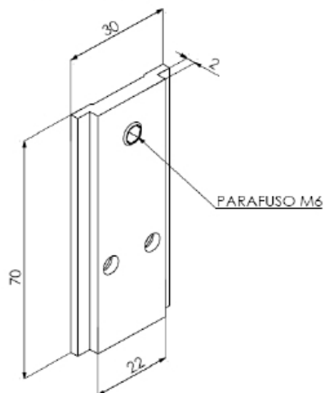
SUP 605 SUPORTE SUPORTE DE FIXAÇÃO DA TRAVA PRETO
