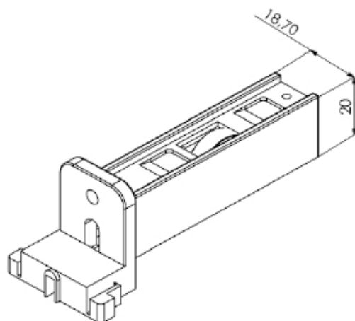
ROL 28.0224 ROLDANA S/ROLAMENTO S/REGULAGEM
