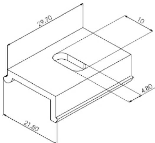
FAA 236 PRESILHA EM ALUMÍNIO
