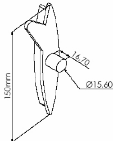
NYL 250 TAMPA NYLON C/ ORELHA ESQUERDA 150 mm
