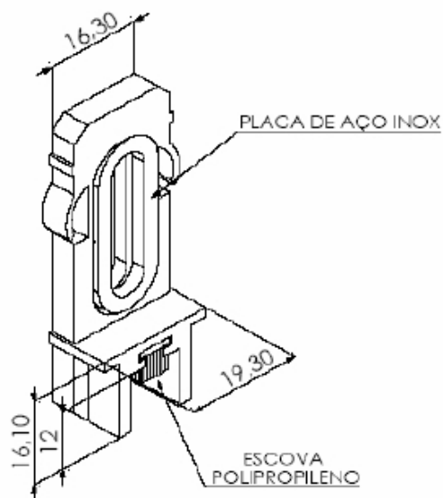
NYL 883 GUIA VEDADOR P/ JANELA
