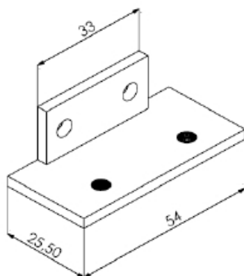
SUP 600 SUPORTE FIXAÇÃO CENTRAL
