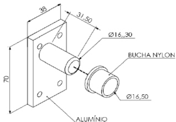
PIV 735 PIVÔT PORTÃO BUZIOS LINHA M.P
