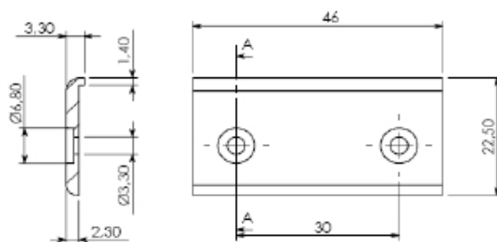
CON 721 CONEXÃO P/ CONTRA MARCO Y - 721
