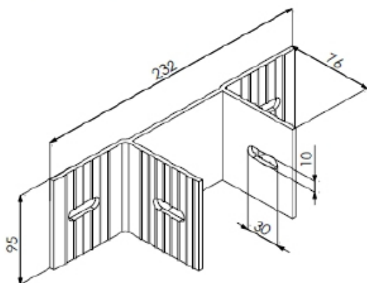
ANC 803 ANCORAGEM CENTRAL LINHA CITTÁ DUE
